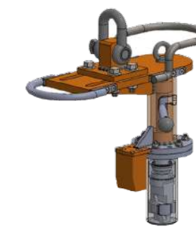
Perno de bloqueo
