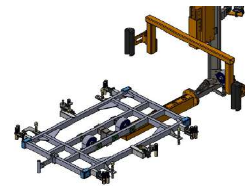
Pernos de localización
