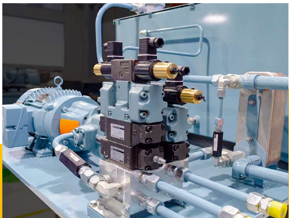
Block hidráulico con válvulas proporcionales para control preciso de flujo y presión
