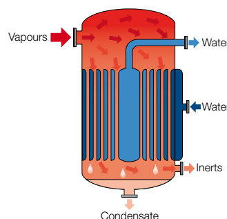
Condenser
