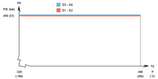
DOC60 – Gráfico de presión/temperatura con homologación UL
