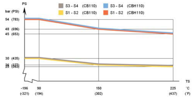
CB110/CBH110– Gráfico de presión/temperatura con homologación UL
