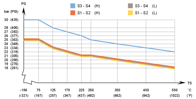
AlfaNova HP 27 - Gráfico de presión/temperatura con homologación PED
