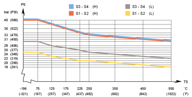
AlfaNova XP27 - Gráfico de presión/temperatura con homologación PED
