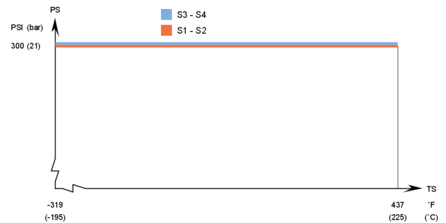
AlfaNova 14 - Gráfico de presión/temperatura con homologación UL
