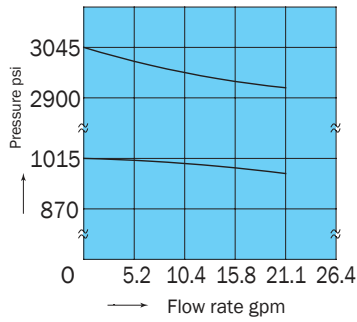
OG-G03-B \frac{1}{3} -J51
