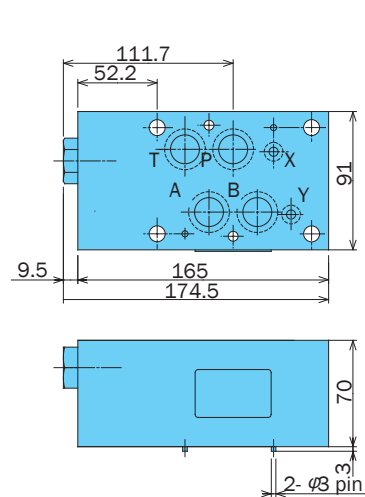
OCH-G04-T*-10
