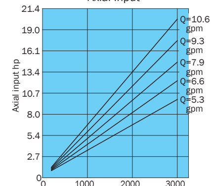
Axial Input
