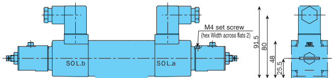
ESD-G03
