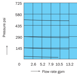
OG-G03-PC-J51
