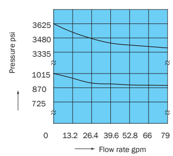
OGH-G04-**-10
