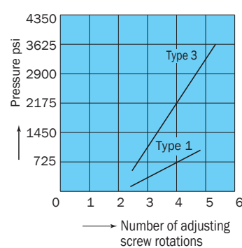
OGH-G04-**-10
