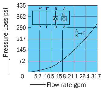
OCP-G03-W*-J50
