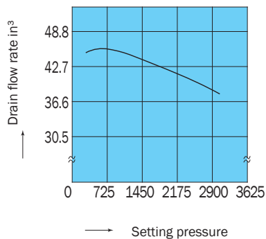
OG-G03-B*-J51
