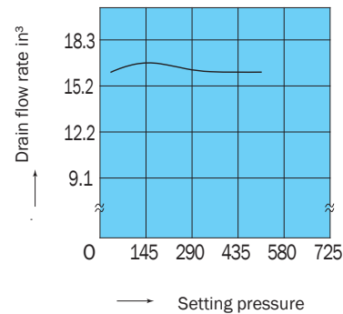
OG-G03-BC-J51
