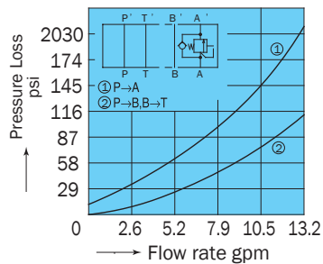
OCQ-G01-A1*-20
