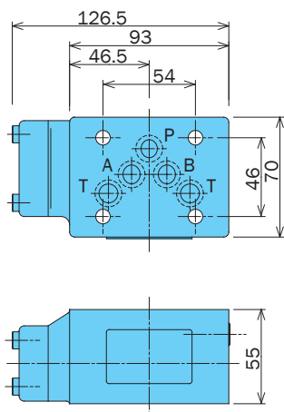
OC-G03- AP
