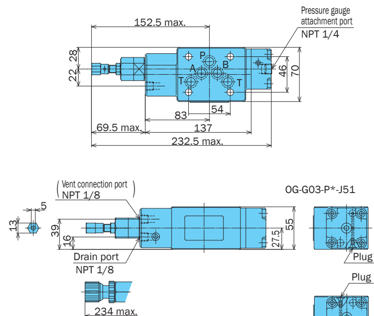
OG-G03-P*-(V)-E51
