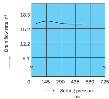
OG-G03-PC-J51
