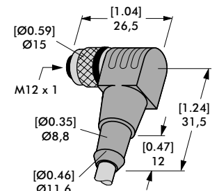
Angular: 8EL-003-1
