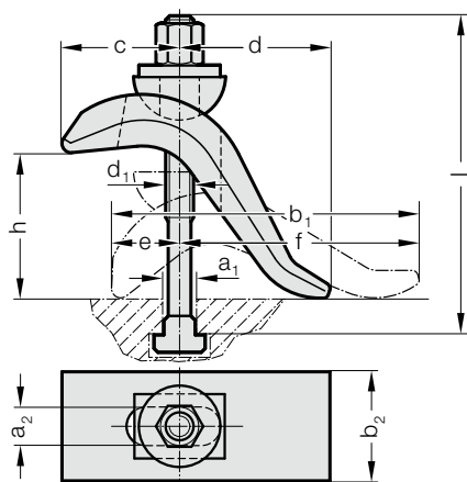
2140.13. Brida, de ajuste gradual
