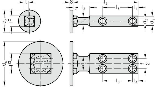
2130.12. Tirante elevador con seguro del cable
