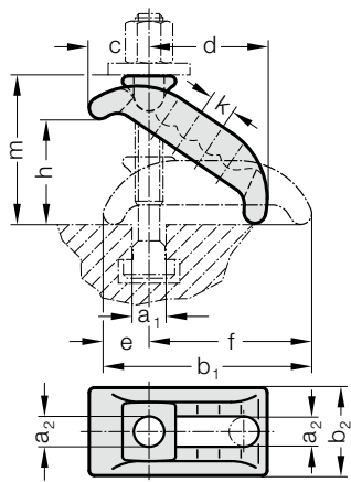
2140.14. Brida, de ajuste gradual
