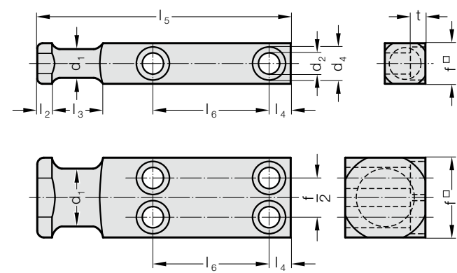
2130.11. Tirante elevador VDI 3366
