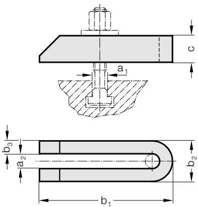
2140.17. Brida de horquilla, con la punta achaflana-da, DIN 6315-B
