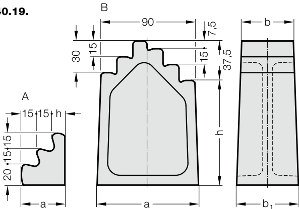
2140.19. Soporte escalonado DIN 6318
