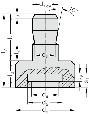
212.16. Perno de acoplamiento con guía
