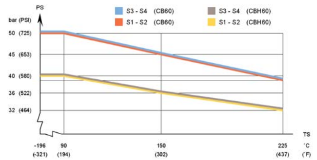
CB60/CBH60 – Gráfico de presión/temperatura con homologación UL
